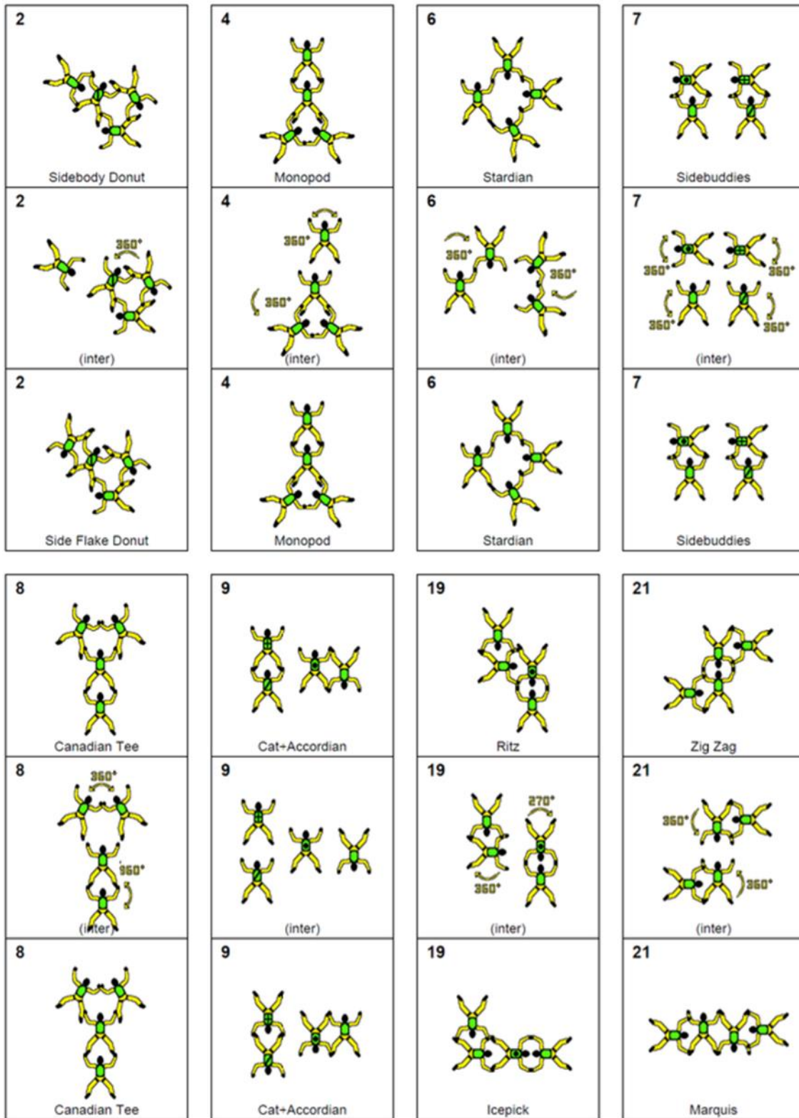
Attachement 2: Blöcke
